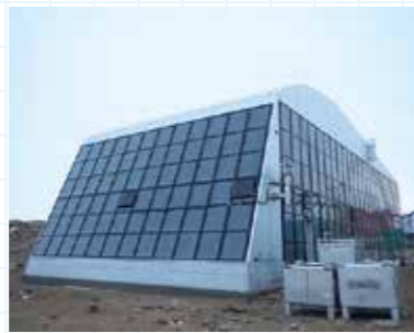
昭和基地・自然エネルギー棟/日本 雪上車など大型車両を整備する建物で、2013年に完成。特徴は太陽光集熱パネルで室内を暖房するシステムを備えていること。これで暖房用の燃料を年間7000 Lも節約できる。
